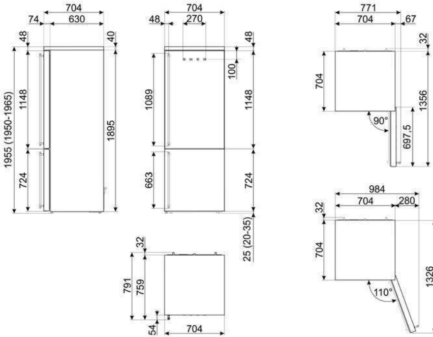
FA8005LAO5/6 ANTRASİT / RUSTİK ESTETİK / SOL MENTEŞE
