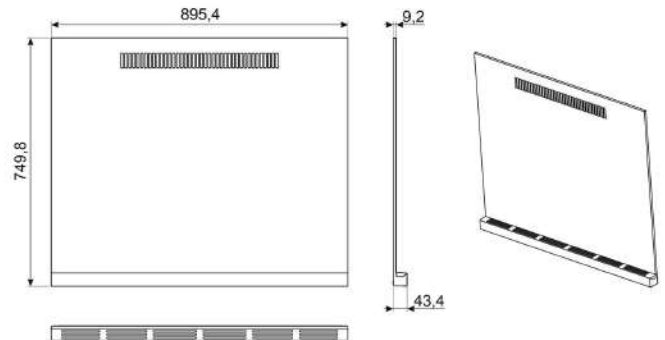
KITPC9X9 (A90G001 serisi opera kuzine için çizim)
