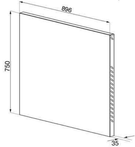
KITPC9X9 (A90G001 serisi opera kuzine için çizim)
